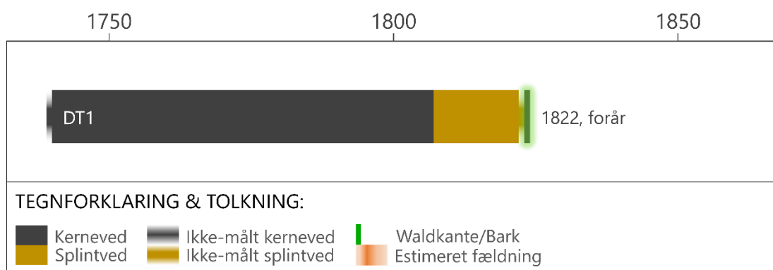
Figur 1: Dateringsdiagram for prøven fra HOM 3923, Nørregade 4 Horsens. Undersøgelsens dateringer placeret på en tidsskala med angivelse af årringssekvensernes længde og konstateret kerneved, splintved, waldkante osv. Evt. beregnede fældningstidspunkter er noteret i forlængelse af prøvernes årringssekvens. Fældningstidspunkter er beregnet vha. splintstatistikker (se evt. Metodebeskrivelse i rapportens bilag); for egetræ 20 [-5+10] årringe i splintved. For prøver med waldkante/bark er det absolutte fældningstidspunkt noteret.
